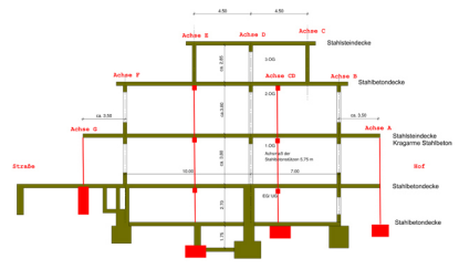
Systemschnitt
